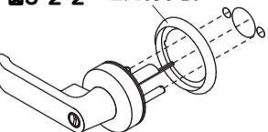
図5-2-2 エスカッション
