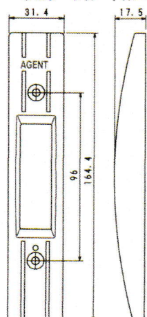
サムターンガードカバー
