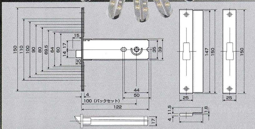
寸法図
